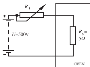
Fig. 1-1: Sturing oven via weerstand
